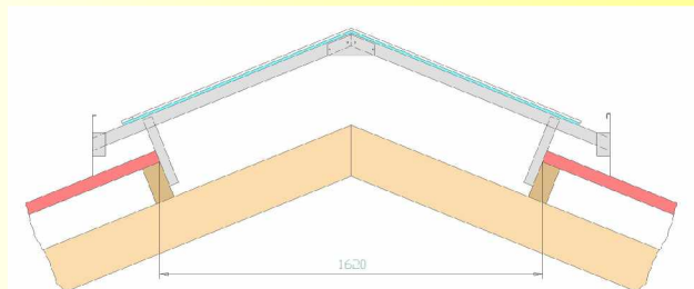
Licht- Lüftungsfirst der Breiten 60, 80, 120 und 162 cm
