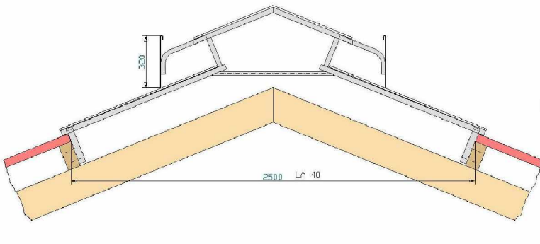
Licht- Lüftungsfirst der Breiten 200 und 250 cm
